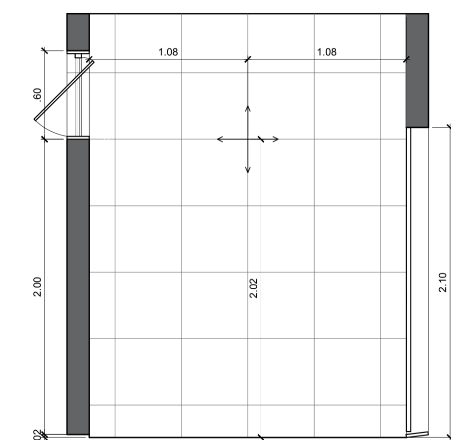
VISTA 2 WC PÚBLICO FEMININO ADAPTADO P/ PNE ESCALA 1:25
