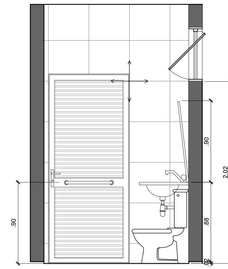
VISTA 4 WC FEMININO PARA FUNCIONÁRIOS ESCALA 1:25
