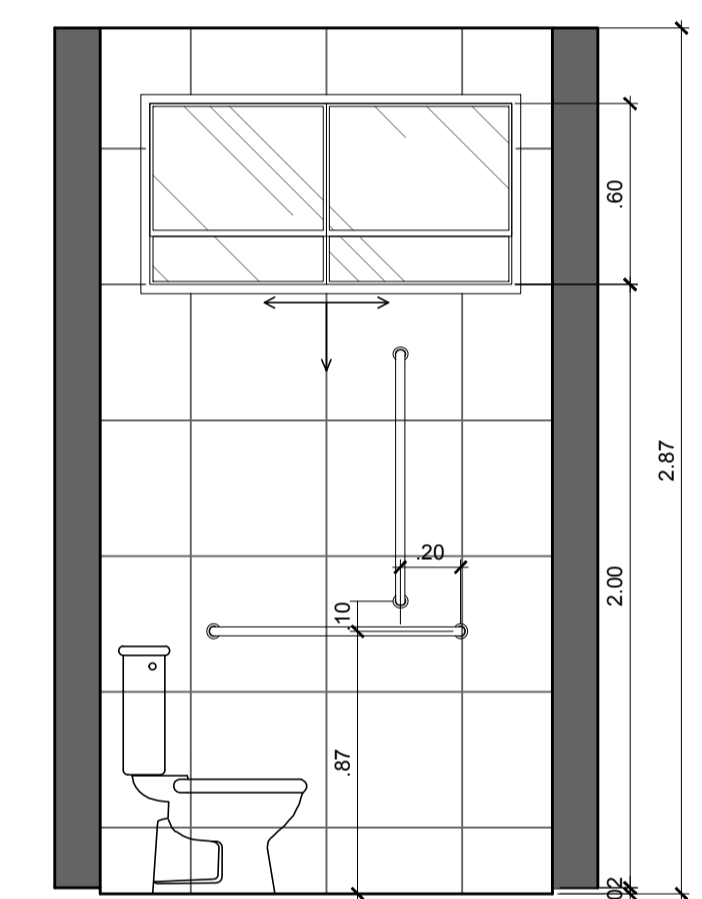
VISTA 1 WC PÚBLICO FEMININO ADAPTADO P/ PNE ESCALA 1:25
