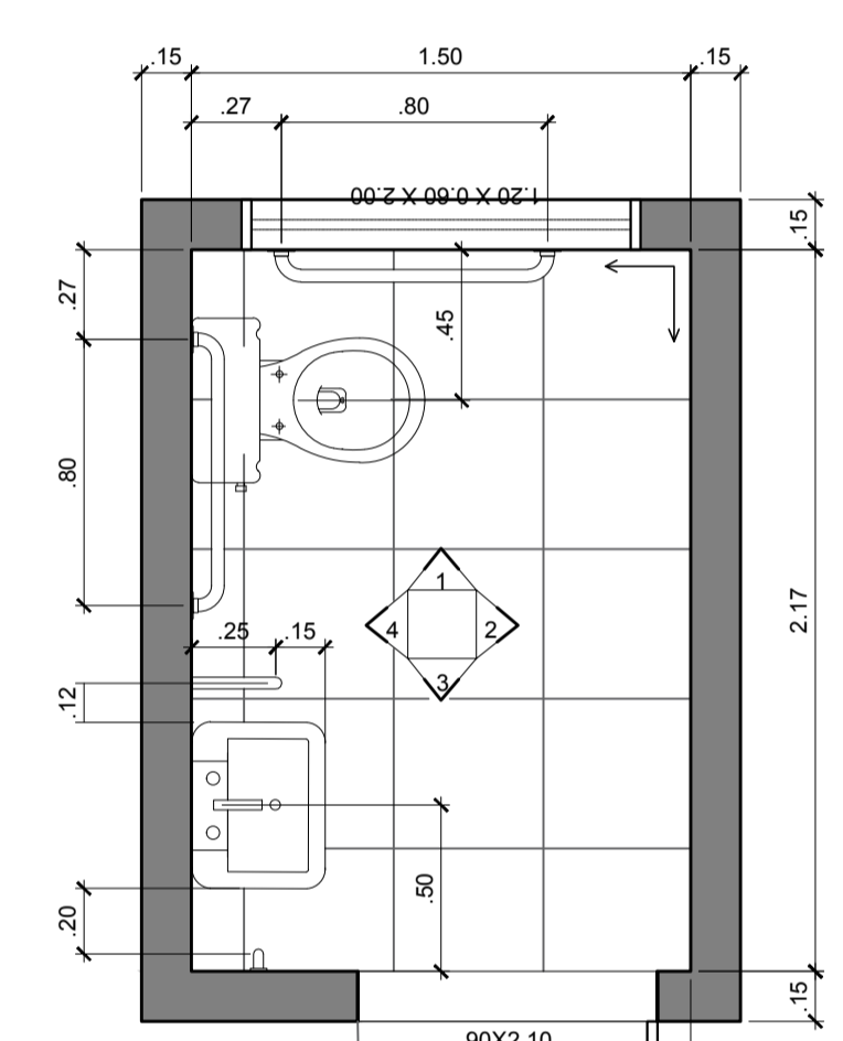
PLANTA BAIXA WC PÚBLICO FEMININO ADAPTADO P/ PNE ESCALA 1:25
