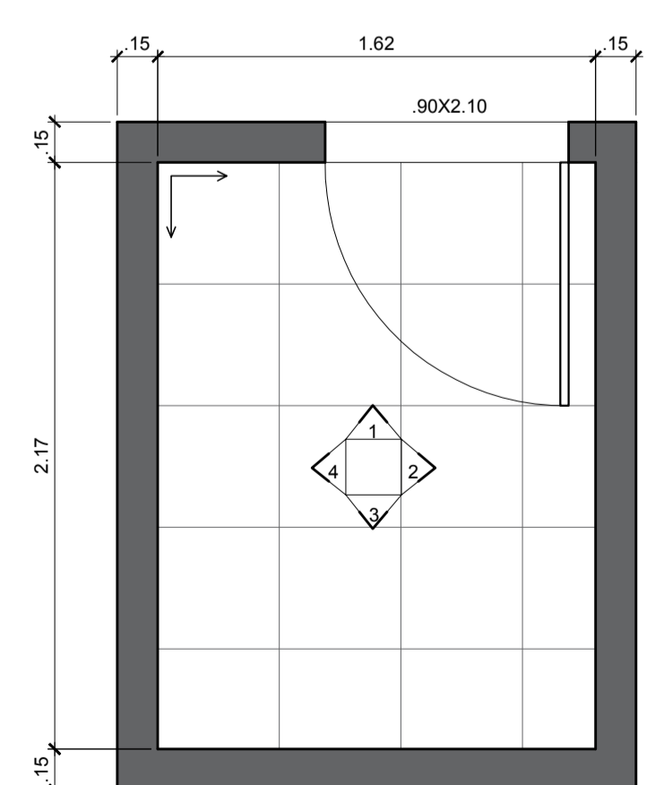
PLANTA BAIXA DEPÓSITO DE RESÍDUOS SÓLIDOS ESCALA 1:25
