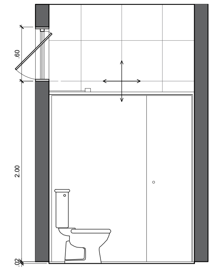
VISTA 2 WC FEMININO PARA FUNCIONÁRIOS ESCALA 1:25
