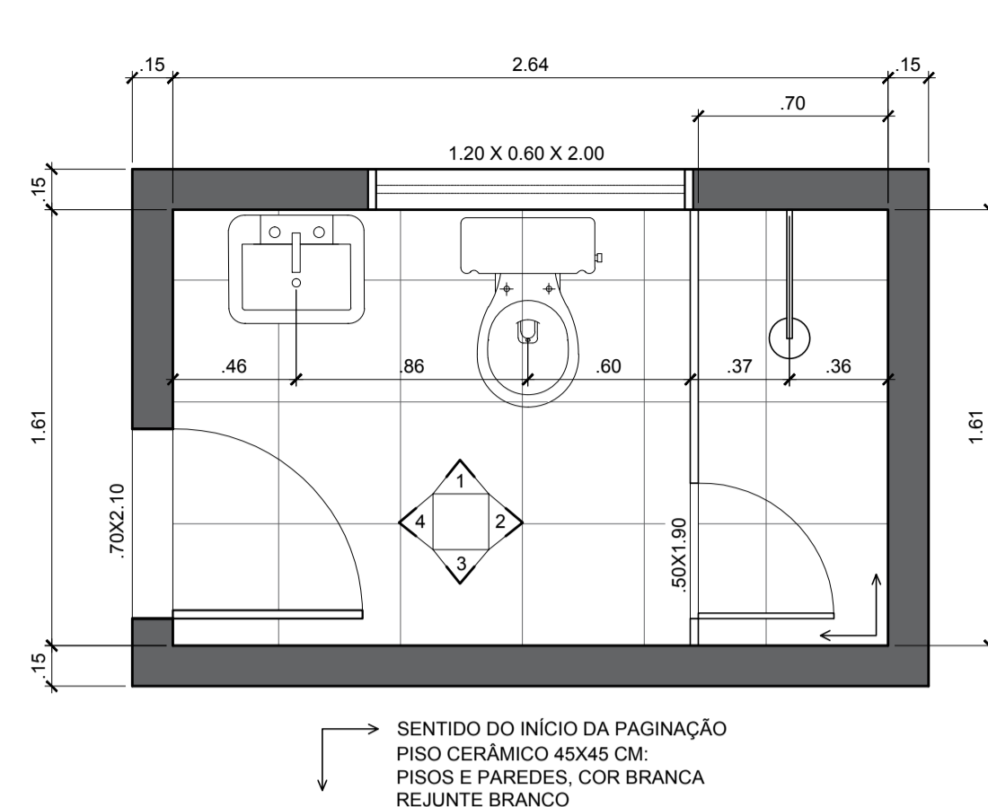
PLANTA BAIXA WC FEMININO PARA FUNCIONÁRIOS ESCALA 1:25
