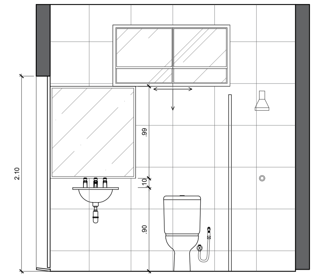
VISTA 1 WC FEMININO PARA FUNCIONÁRIOS ESCALA 1:25
