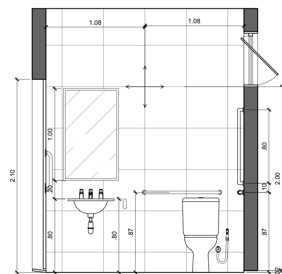
VISTA 4 WC PÚBLICO FEMININO ADAPTADO P/ PNE ESCALA 1:25
