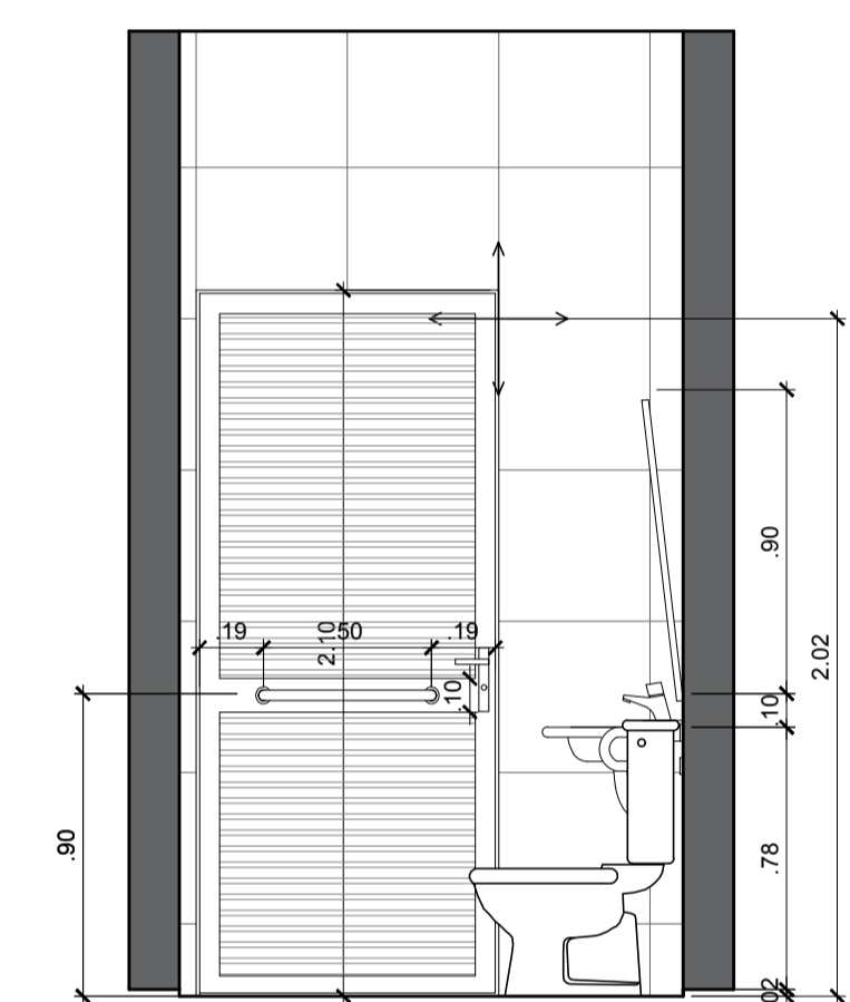
VISTA 3 WC PÚBLICO FEMININO ADAPTADO P/ PNE ESCALA 1:25
