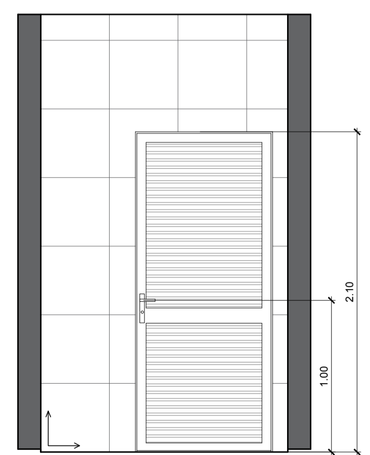
VISTA 1 DEPÓSITO DE RESÍDUOS SÓLIDOS ESCALA 1:25
